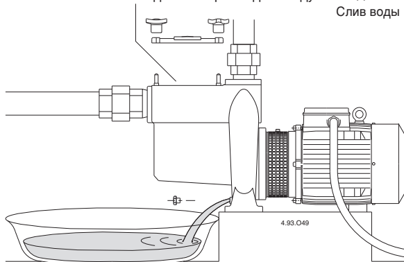
FIG. 3 Scarico Draining Entleerung Entleerung Vidange Vaciado Dränering Aftappen Слив воды
