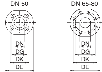
Flanges in accordance EN 1092-2 PN 25 - 40
